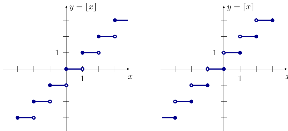
Figure 3.5 – Graphes des fonctions y = [x] (partie entière inférieure) et y = \lceil x \rceil (partie entière supérieure).
