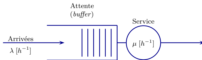
Figure 4.2 – Représentation schématique du serveur de calcul de l'exercice 4.80.
